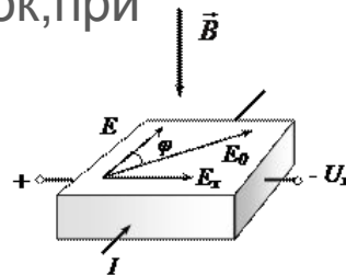
Рис. 8.1.1. Эффект Холла
